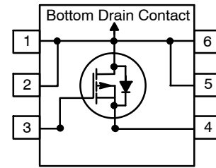
P-Channel MOSFET
