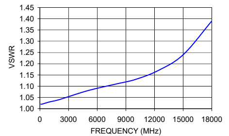
BW-S7W2+ VSWR
